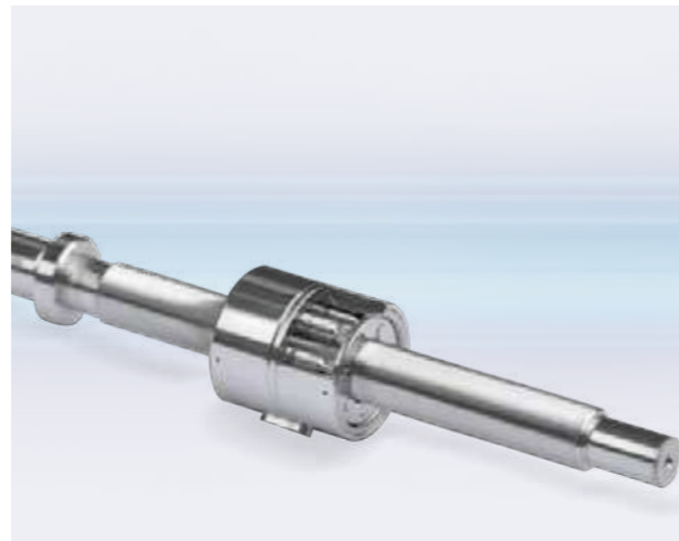
ROLLENGEWINDETRIBE
